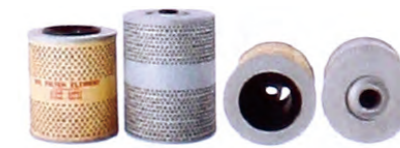
FYT1164 HENGST: MAN: OEM:31240-53053/53054
